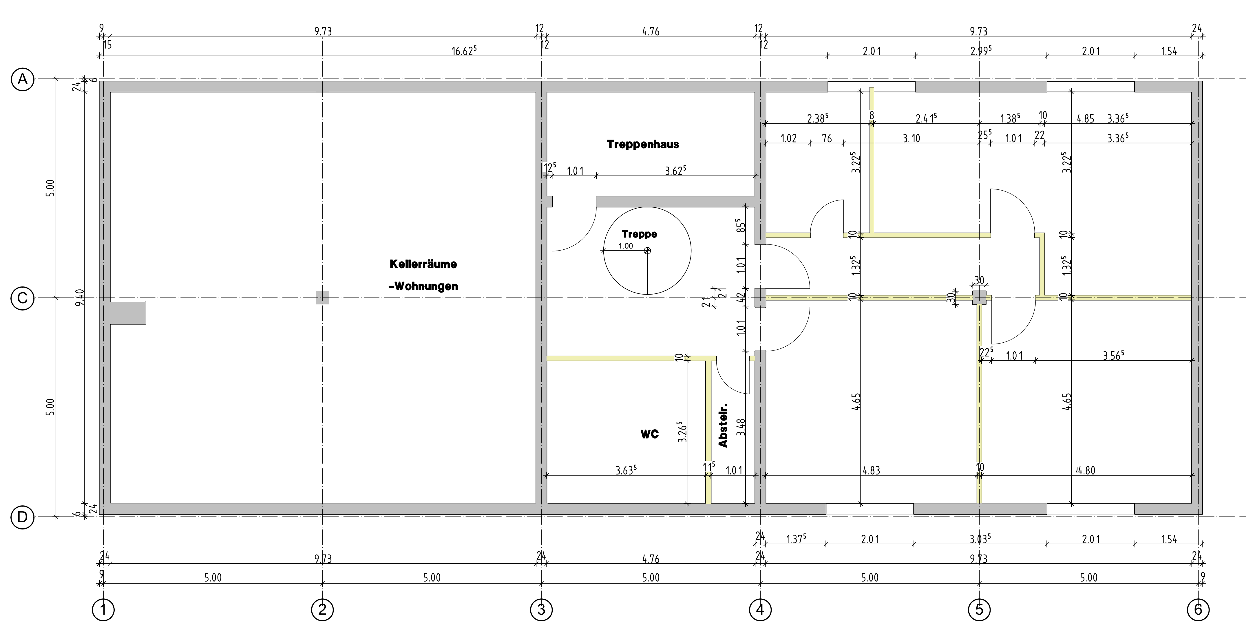
Kellergeschoss M.1:50
