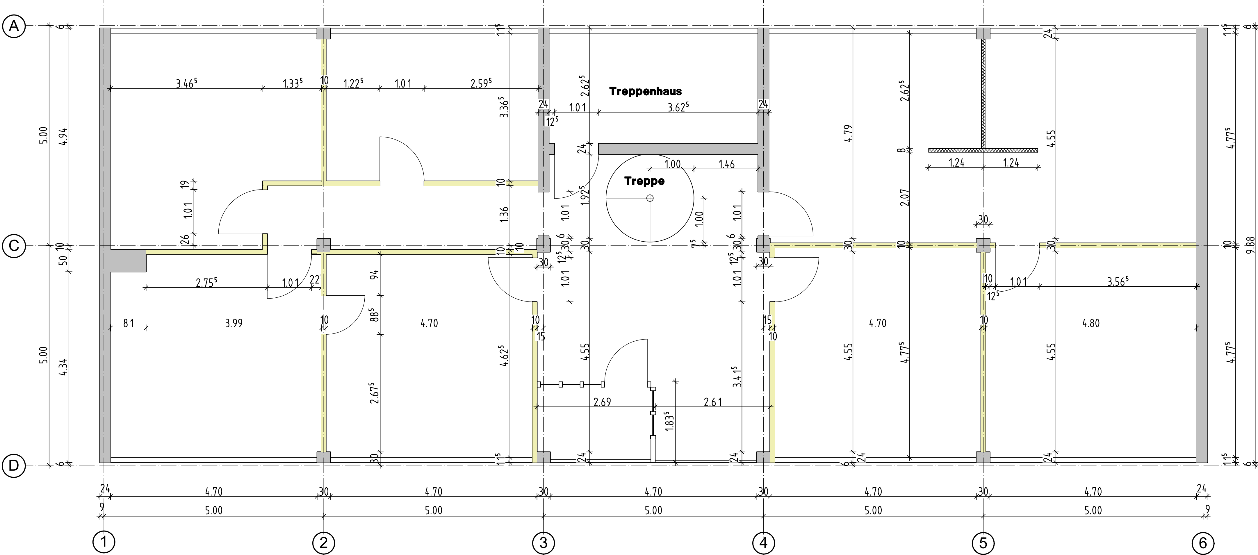
Erdgeschoss M.1:50
